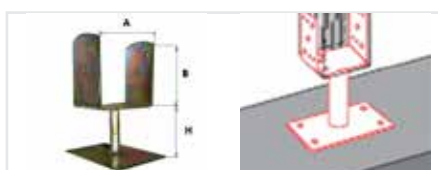
Suport grindă formă U cu tijă și talpă
