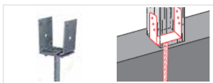
Suport grindă formă URT reglabil pe lățime, cu tijă
