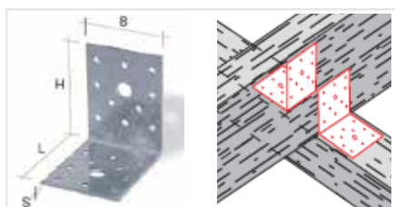
Colțar metalic
