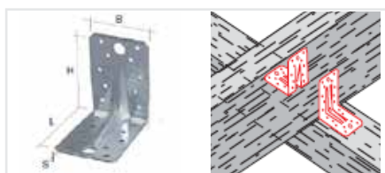
Colțar metalic cu nervură
