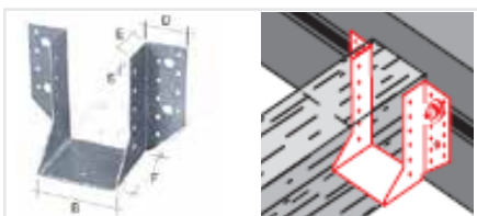
Reazem grindă exterior
