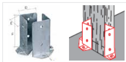
Suport pătrat / 2
