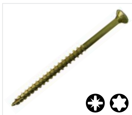
Șurub pentru lemn, cap înecat, filet parțial, filet cu 2 începuturi tip DNS
