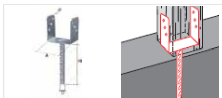
Suport grindă formă UT cu tijă
