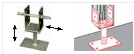
Suport grindă reglabil UrVH pe lățime și înălțime
