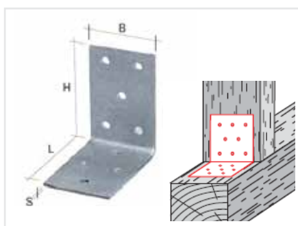
Vinclu din placă perforată
