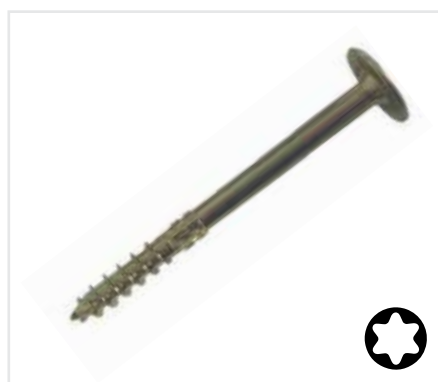
Șuruburi pentru construcții din lemn cu cap plat tip șaiabă, amprentă Torx
